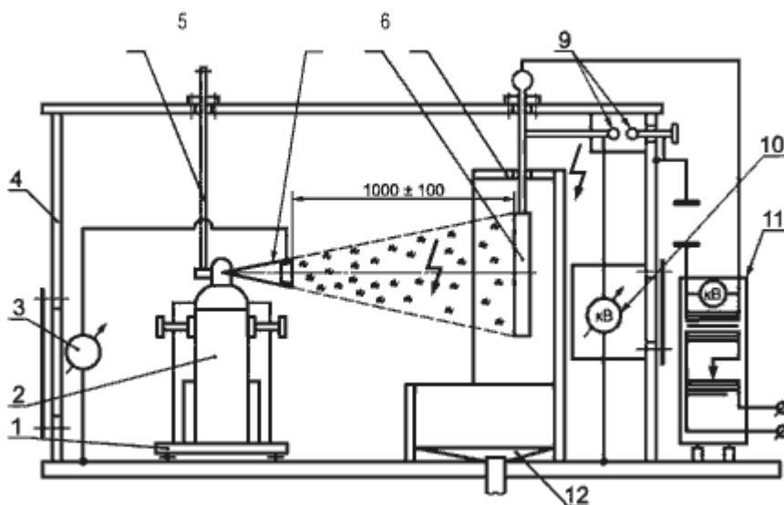
1-изолирующая подставка; 2-испытываемый огнетушитель; 3-измеритель тока утечки; 4-защитный каркас испытательного стенда; 5-устройство запуска огнетушителя; 6-насадок огнетушителя с электропроводным элементом; 7-мишень; 8-экран; 9-разрядник;
