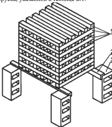
Рисунок Б.1 — Устройство деревянного штабеля (модельного очага пожара класса А) для проведения огневых испытаний
